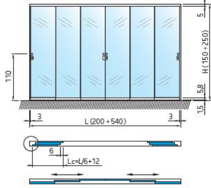
3-way - 6 door version
