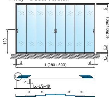
4-way - 8 door version
